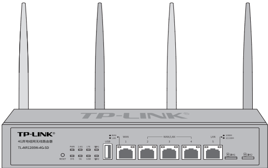
图1-1 前面板示意图
