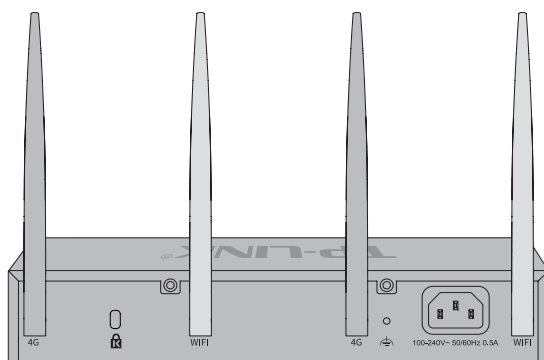
图1-2 后面板示意图
