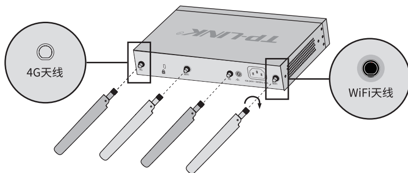
图2-3 产品安装天线示意图
